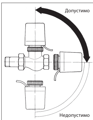
Допустимое монтажное положение запорного клапана с термоэлектрическим сервоприводом
